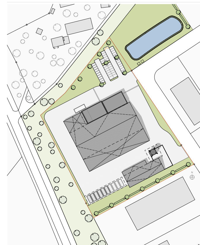
Lageplan | Straßenmeisterei Goslar S3 Sasse + Sasse GmbH
